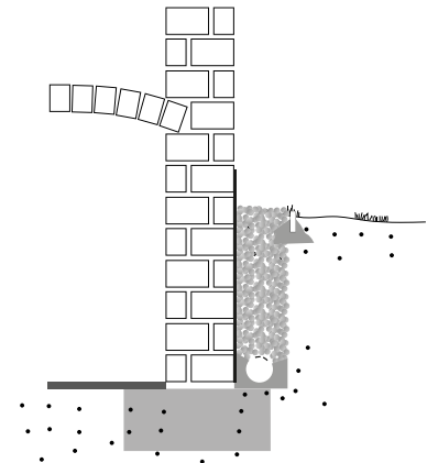
Abdichtung von aussen
