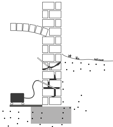
Injektion von Rissen und Hohlstellen
