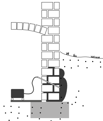
Schleierinjektion
