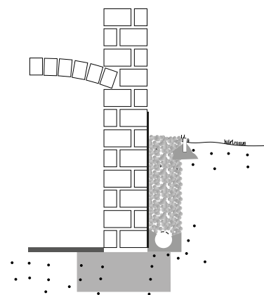
Etanchéification par l'extérieur
