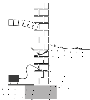
Injection dans les fissures et les cavités
